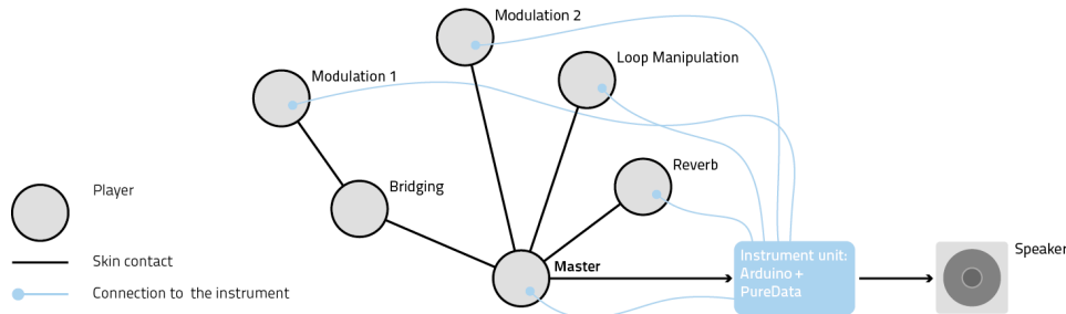
Abbildung 2: Schematischer Aufbau des Prototyps
